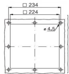
安装开孔图 Cut-out
