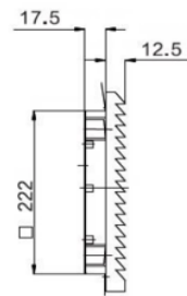
侧视图(出口) Side View (Outlet)
